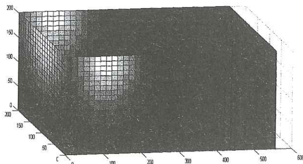
Figura 6 Distribuția nivelului de iluminare pe pereții laterali
